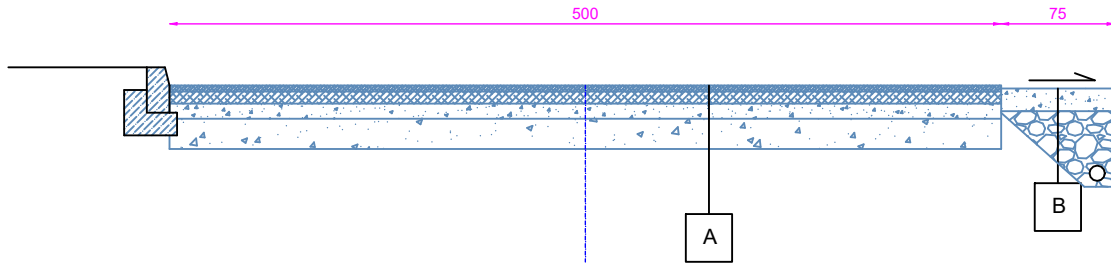
PRZEKRÓJ -B-
